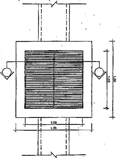
ฉายแปลนเปิดพักน้ำ
