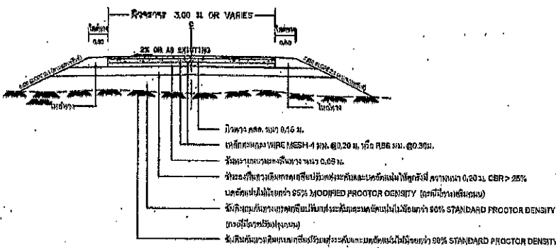
รูปตัดหน้าผิวจราจรก่อนการขึ้นผิวจราจร
